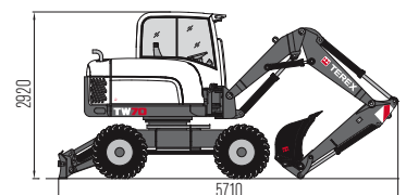
Abb. 3: Transportstellung
