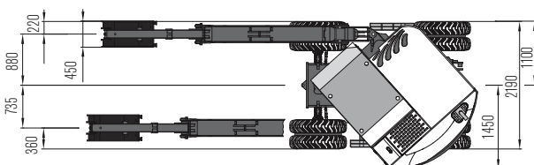
Abb. 1: Spurdeckendes Baggern
